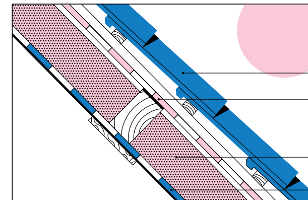
fig. 1 Dakisolatie bij hellende daken geplaatst aan de binnenzijde
