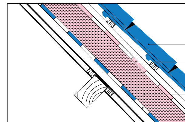
fig. 2 Dakisolatie bij hellende daken geplaatst aan de buitenzijde (sarking-methode)
