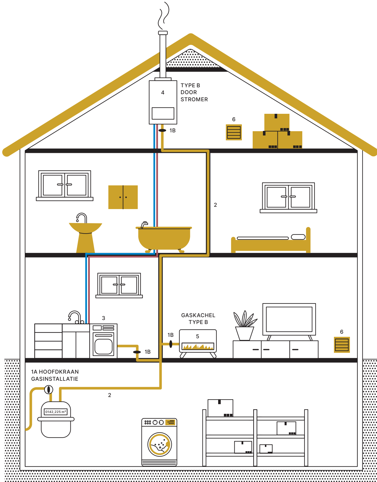
fig 1 Vereisten voor verbrandingstoestellen
