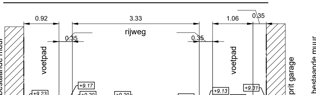
TYPE DWARSPROFIEL 12-12 school 1/50
