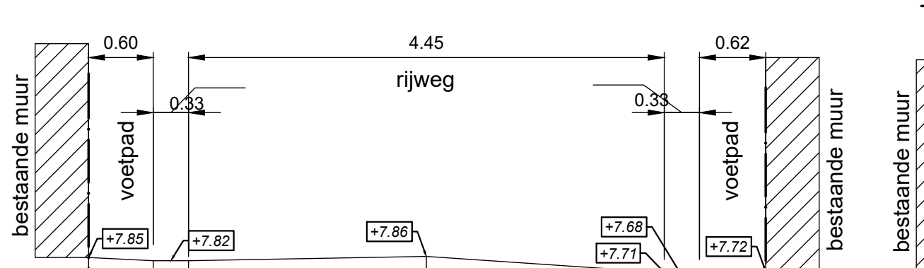
TYPE DWARSPROFIEL 9-9 school 1/50
