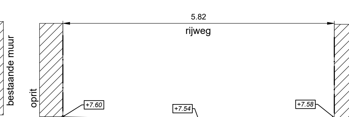
TYPE DWARSPROFIEL 6-6 school 1/50
