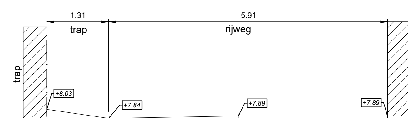
TYPE DWARSPROFIEL 5-5 school 1/50
