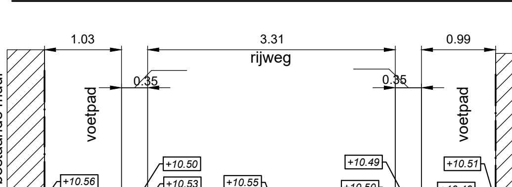
TYPE DWARSPROFIEL 13-13 school 1/50
