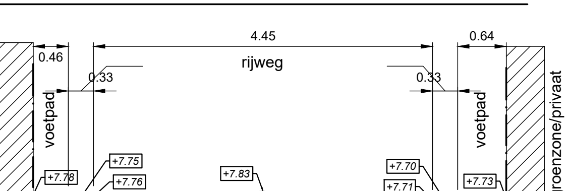
TYPE DWARSPROFIEL 10-10 school 1/50
